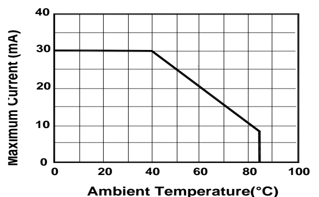
8).Thermal Design
