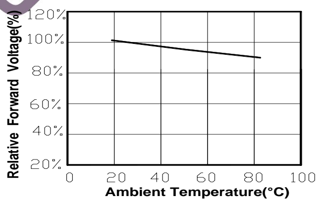
8).Thermal Design
